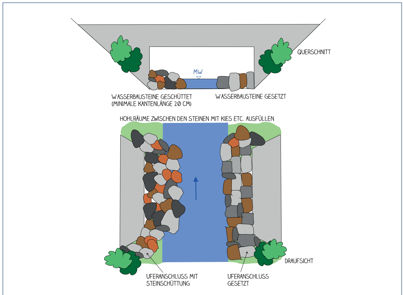
ABB. 6: MERKMALE VON BERMEN AUS WASSERBAUSTEINEN (GRAFIK M. SCHMALZ)
