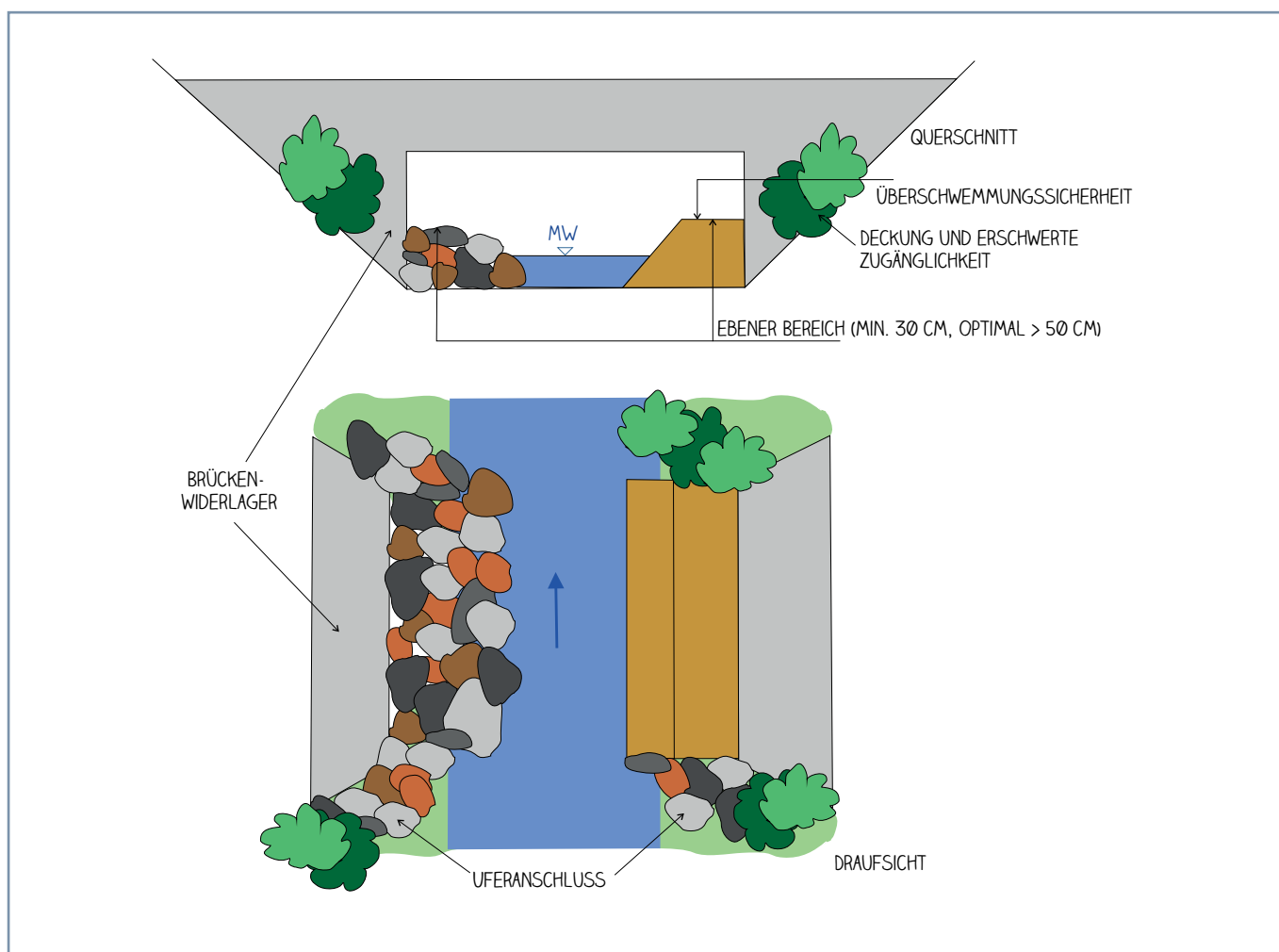
ABB. 5: MERKMALE OPTIMALER BERMEN (GRAFIK M. SCHMALZ)
