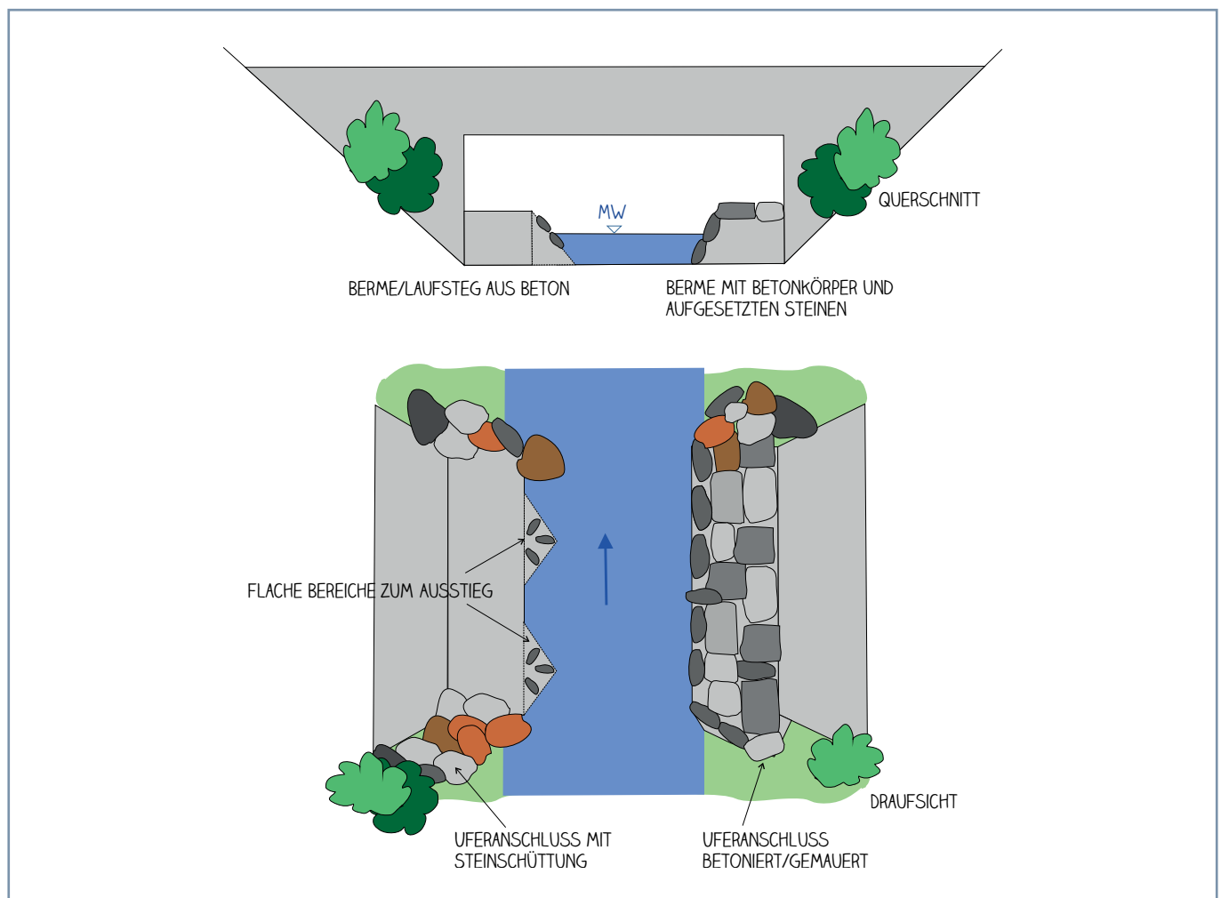
ABB. 11: MERKMALE VON BERMEN AUS BETON (GRAFIK M. SCHMALZ)
