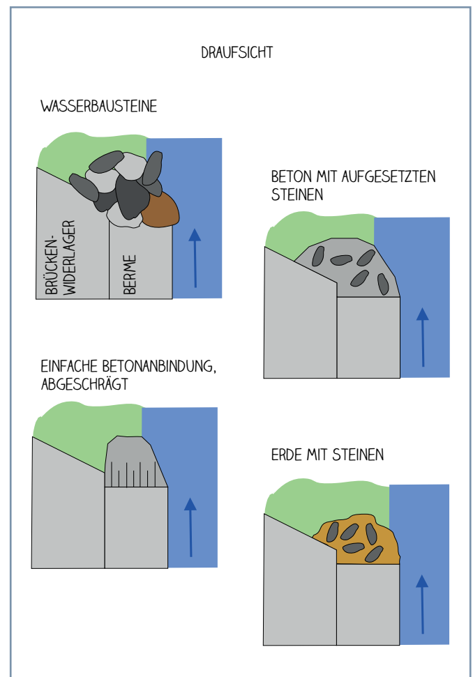
Abb. 35: VERSCHIEDENE MÖGLICHKEITEN DES UFERANSCHLUSSES DER BERMEN (GRAFIK M. SCHMALZ)
